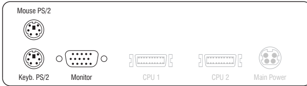
Abbildung 2: Schnittstellen zum Anschluss der Geräte des Arbeitsplatzes
