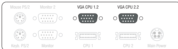
Abbildung 5: Schnittstellen zum Anschluss von »Videokanal 2« beider Rechner
